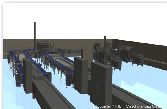
Rendering einer Anlage zum Schneiden von Frischfleisch, beispielsweise Nackensteaks
