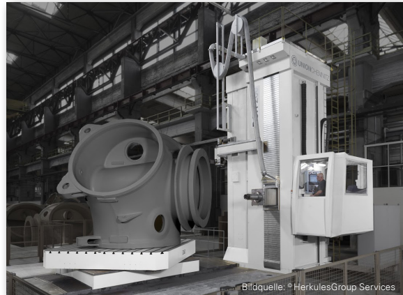
Bearbeitung einer riesigen Rotornabe eines Windrades mit einem UnionChemnitz Bohrerwerk
