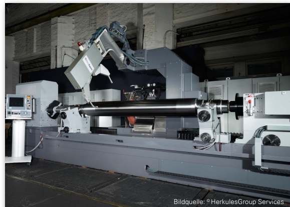
Modernste Technologie Walzenschleifmaschine der Maschinenfabrik Herkules
